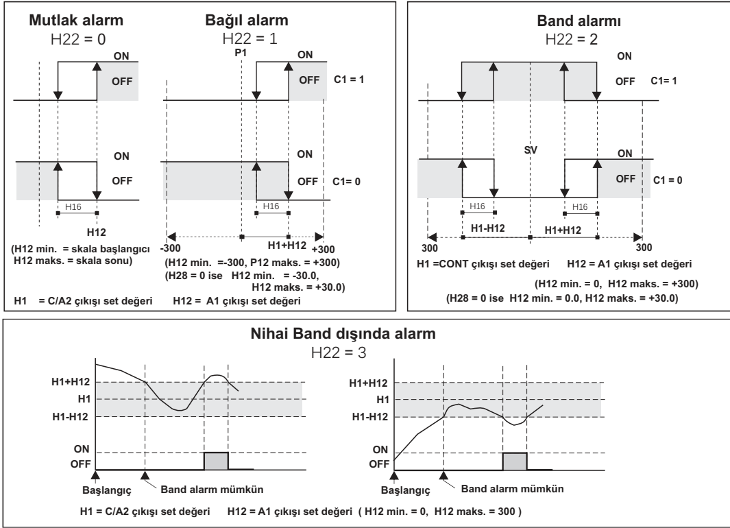
Şekil.1 ALARM1 VE ALARM2 ÇIKIŞ BIÇİMLERİ (Diyagramlar Alarm1 için düzenlenmiştir)
